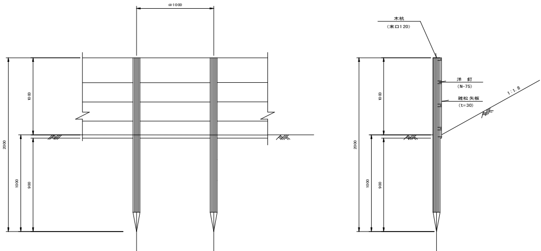
板 柵 工 S=1:25
