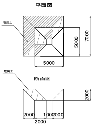
3号調整池東側沈砂池 埋戻図 S=1:200
