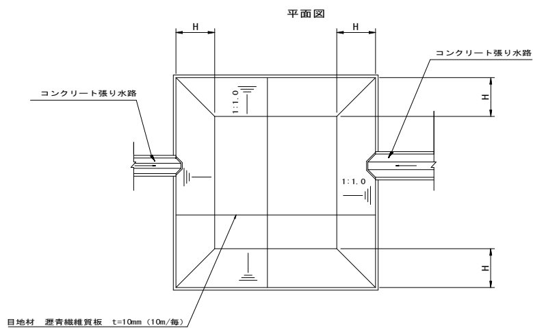
コンクリート張沈砂池 S=1:200
