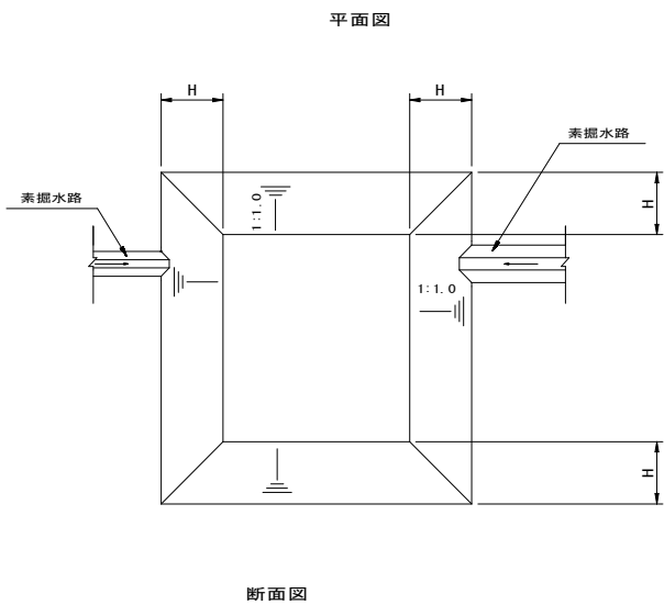
素掘沈砂池 S=1:200
