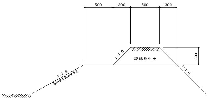
防災小堤 S=1:20
